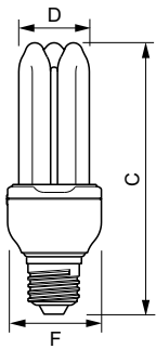
GENIE 18W CDL E27 220-240V 1PF/6
